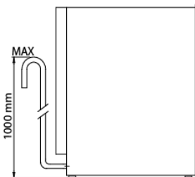
DRAIN PUMP MODELS MODELLI POMPA SCARICO ABLAUFpumpe MODELLE MODELES POMPE DE VIDANGE MODELO DE BOMBA DE DRENAJE
